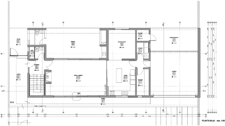
PLANTA BAJA - esc. 1:50
