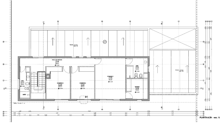
PLANTA ALTA - esc. 1:50
