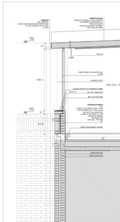
DETALLE 1 esc:1/20
