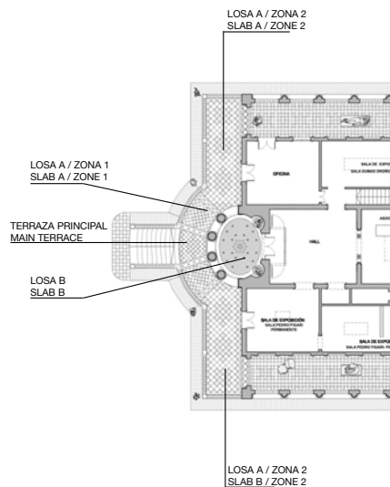
PLANTA PRINCIPAL ZONA DE ACCESO ACCESS ZONE
