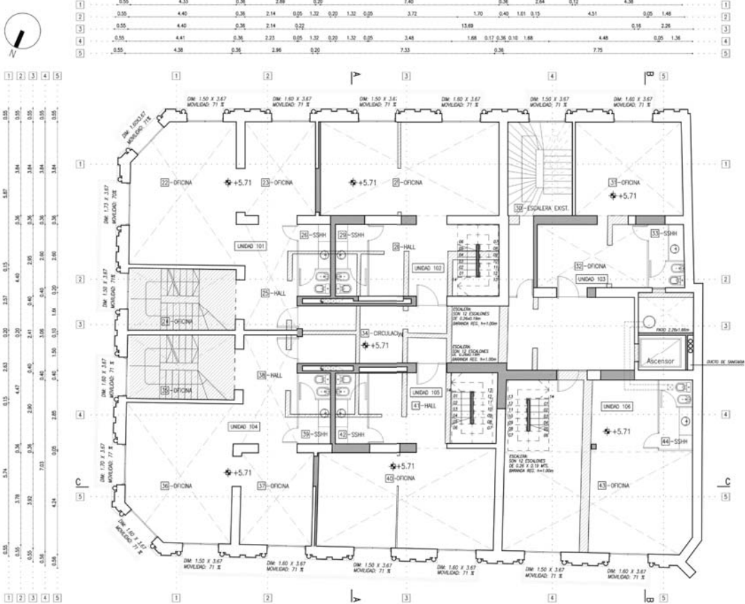
PLANTA NIVEL +5.71/+10.76
